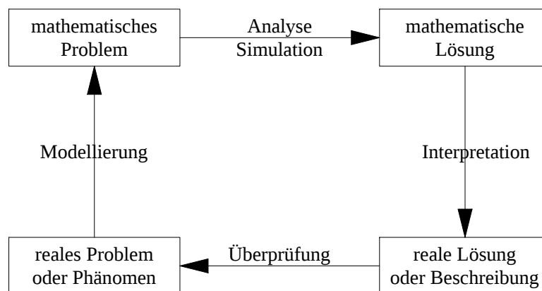
Abbildung 2: Der Modellierungsprozess
